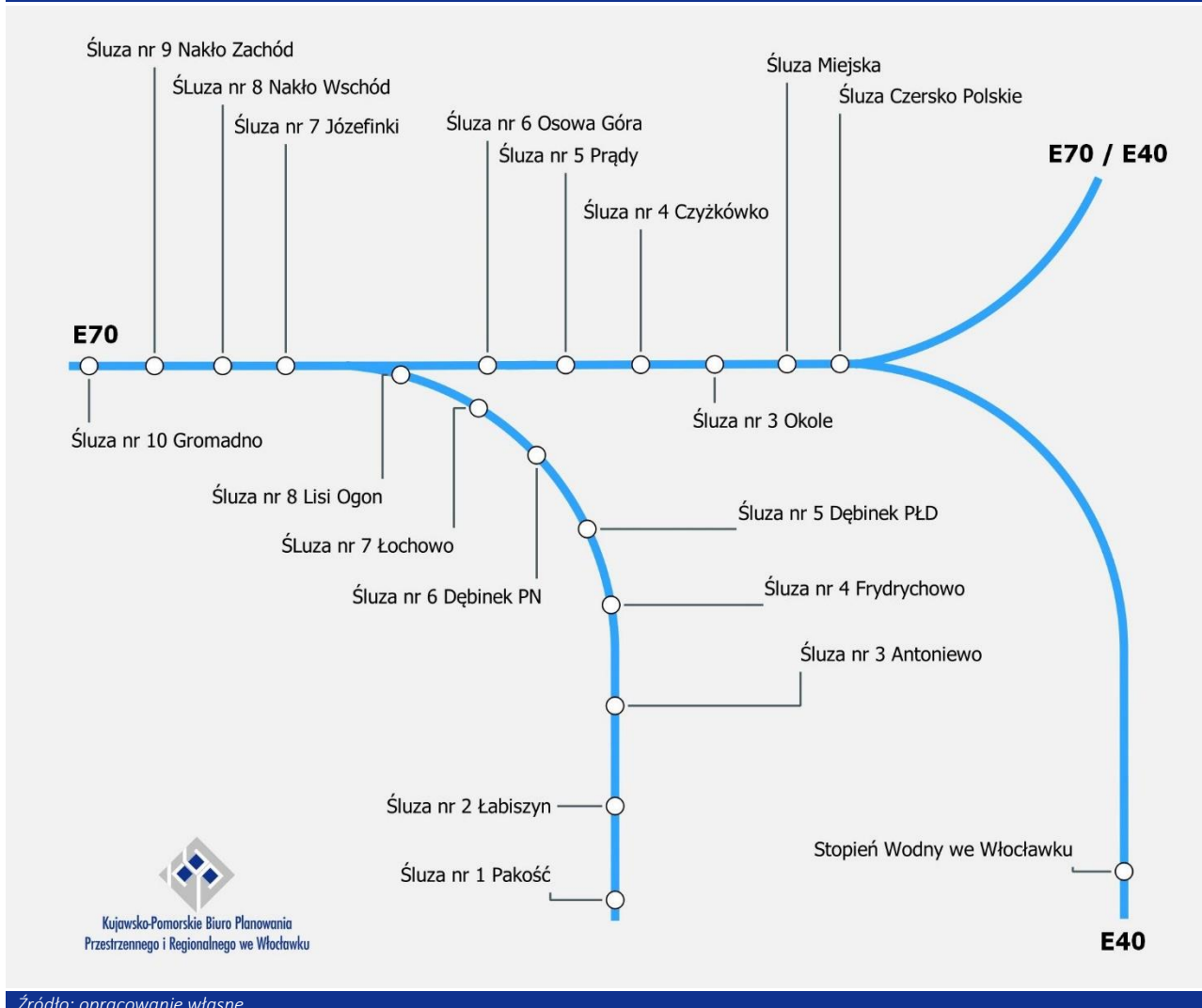
Schemat 1. Śródlądowe drogi wodne wraz ze śluzami żegludowymi
