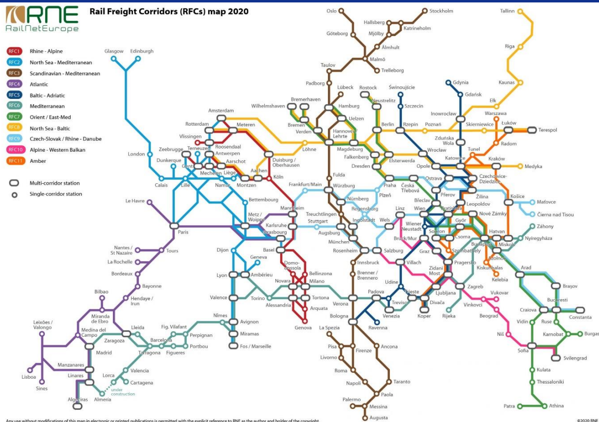
Mapa 24. Schemat sieci w ramach RFC
